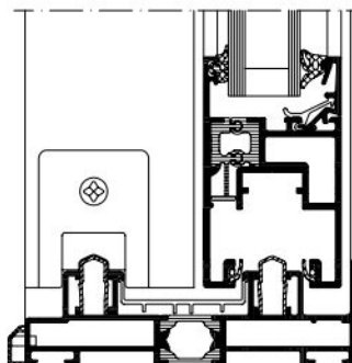
AluClear Schiebesystem ASS 50, Maßstab 1:3 AluClear ASS 50 sliding system, scale 1:3
